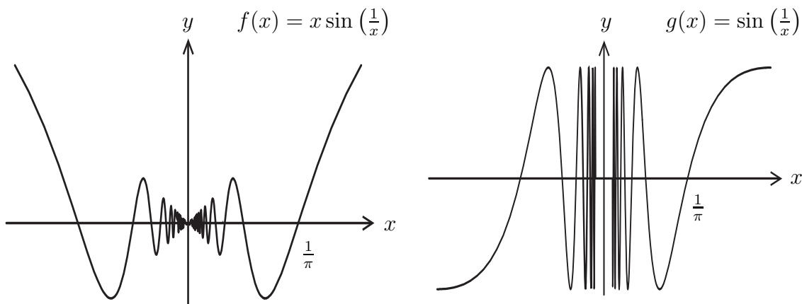
圖 4.2: 函數 f(x) = x \sin\left(\frac{1}{x}\right) 與 g(x) = \sin\left(\frac{1}{x}\right) 的圖形, 兩函數的圖形在 x = 0 附近皆無法確實描繪。
