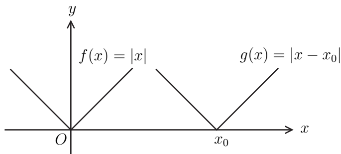
圖 4.3: 將函數 f(x) = |x| 的圖形向右平移 x_0 單位則為函數 g(x) = |x - x_0| 的圖形。
