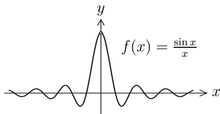
圖 4.1: 函數 f(x) = \frac{\sin x}{x} 的圖形在趨近於正、負無窮時有水平漸近線 y = 0 。
